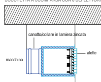
SEZIONE VERTICALE CON VISTA LATERALE DEL BOCCHETTA A SCOMPARSA CON 6 DEFFLETTORI
