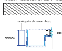
SEZIONE VERTICALE CON VISTA LATERALE DEL DIFFUSORE A SCOMPARSA CON 3 DEFFLETTORI
