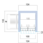
Dettaglio PSBVMC con attacco S
