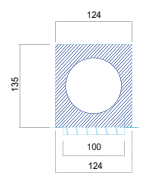
Dettaglio PSBVMC con attacco L
