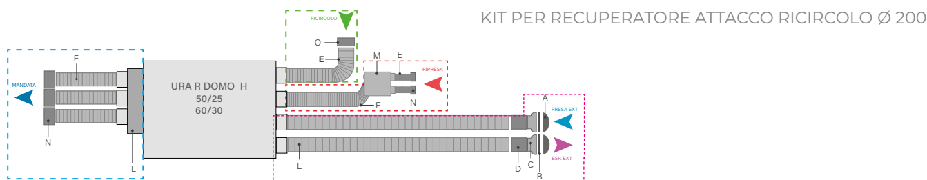
COMPONENTI KIT
