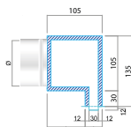
Dettaglio PSFVMC con attacco S
