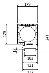
ATTACCO LATERALE*
