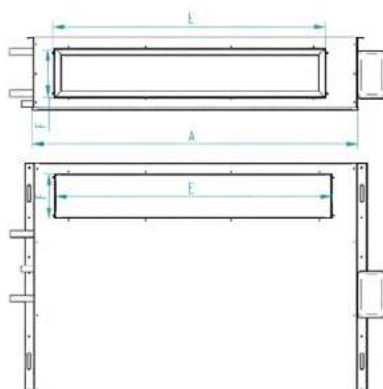
CANALE RETTANGOLARE
