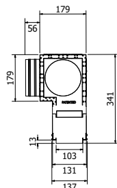
ATTACCO SUPERIORE
