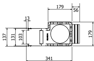
ATTACCO POSTERIORE
