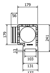
ATTACCO SUPERIORE
