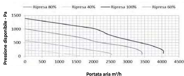
LATO ESPULSIONE
