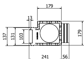
ATTACCO POSTERIORE
