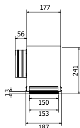
ATTACCO SUPERIORE
