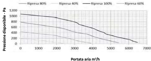
LATO ESPULSIONE
