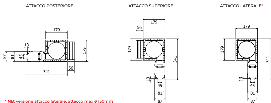
DIMENSIONALI PSF H40 - INSTALLAZIONE MURO
