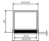
plenum MANDATA/RIPRESA altezza 200 mm
