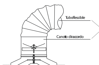
Montaggio con tubo flessibile
