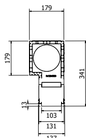
ATTACCO LATERALE*
