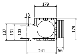
ATTACCO POSTERIORE
