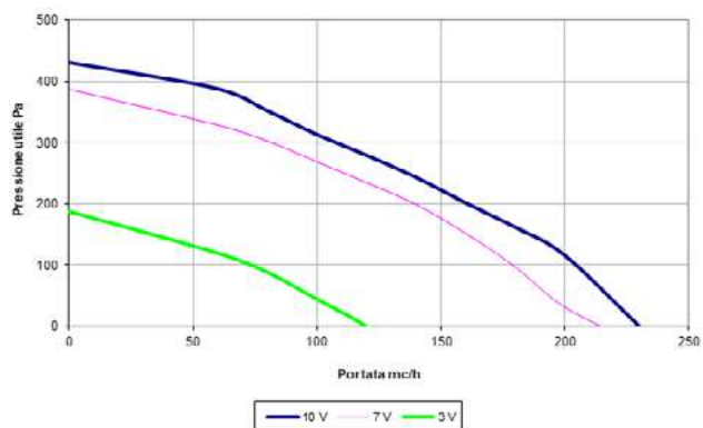
URC DOMO SMART 20Z
