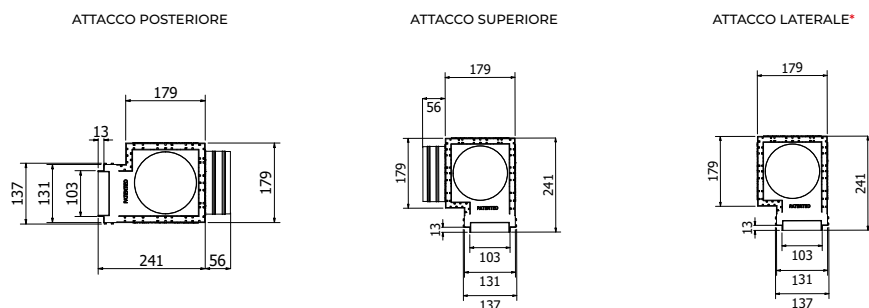
DIMENSIONALI PSB H100 - INSTALLAZIONE CARTONGESSO
