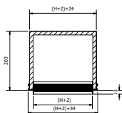
plenum attacco laterale altezza 200 mm
