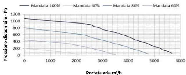
LATO RINNOVO
