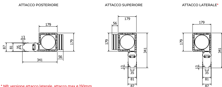
DIMENSIONALI PSF H30 - INSTALLAZIONE MURO
