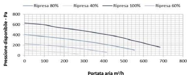
LATO ESPULSIONE
