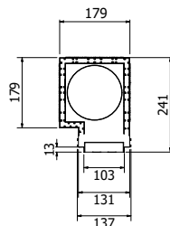
ATTACCO LATERALE*
