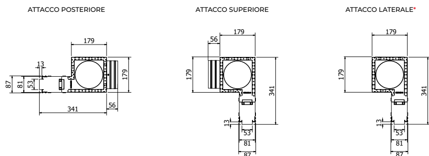
DIMENSIONALI PS2F H50 - INSTALLAZIONE MURO
