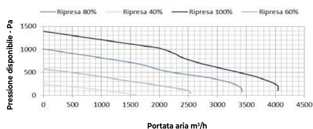
LATO ESPULSIONE
