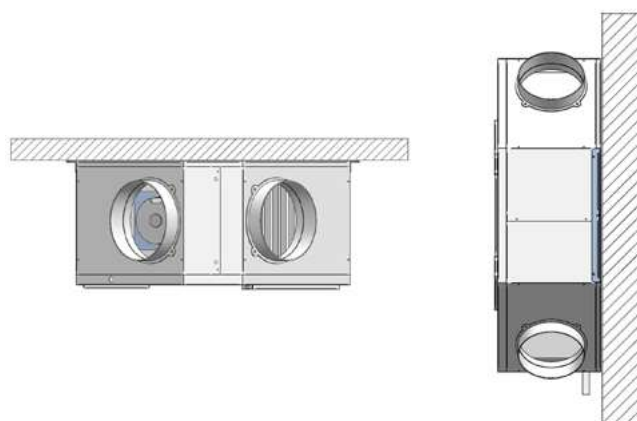
TIPOLOGIA INSTALLAZIONE
