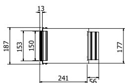
ATTACCO POSTERIORE
