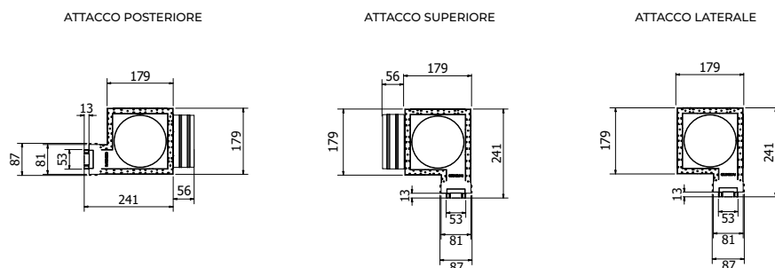
DIMENSIONALI PSD H50 - INSTALLAZIONE CARTONGESSO
