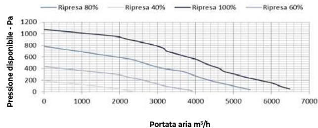
LATO ESPULSIONE
