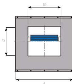
VISTA FRONTALE
