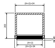
plenum MANDATA/RIPRESA altezza 200 mm
