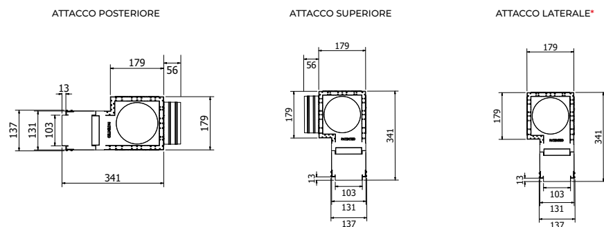
DIMENSIONALI PSB H100 - INSTALLAZIONE MURO
