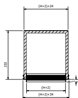
plenum attacco superiore altezza 100 mm
