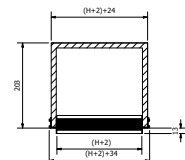
plenum MANDATA/RIPRESA altezza 100 mm
