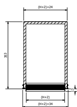
plenum attacco laterale altezza 100 mm
