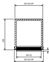
plenum attacco superiore altezza 200 mm
