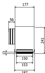
ATTACCO SUPERIORE
