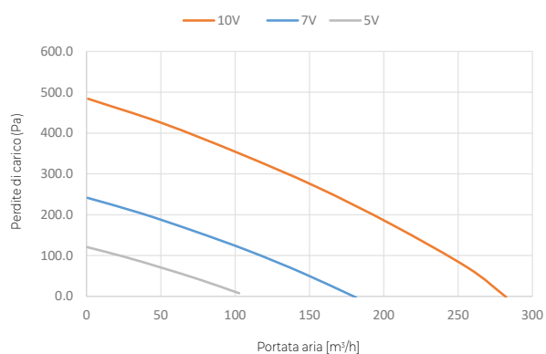
URC DOMO SMART 20V
